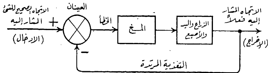
شكل ( ٦ ) شكل بلوكات لنظام تحكى يتضمن الاشارة بالاصبع الى شىء ( متحرك أو ثابت ) .
